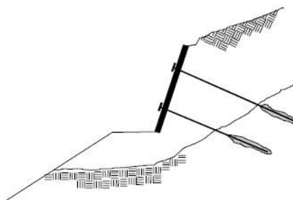
(ب) پایدارسازی شیب
