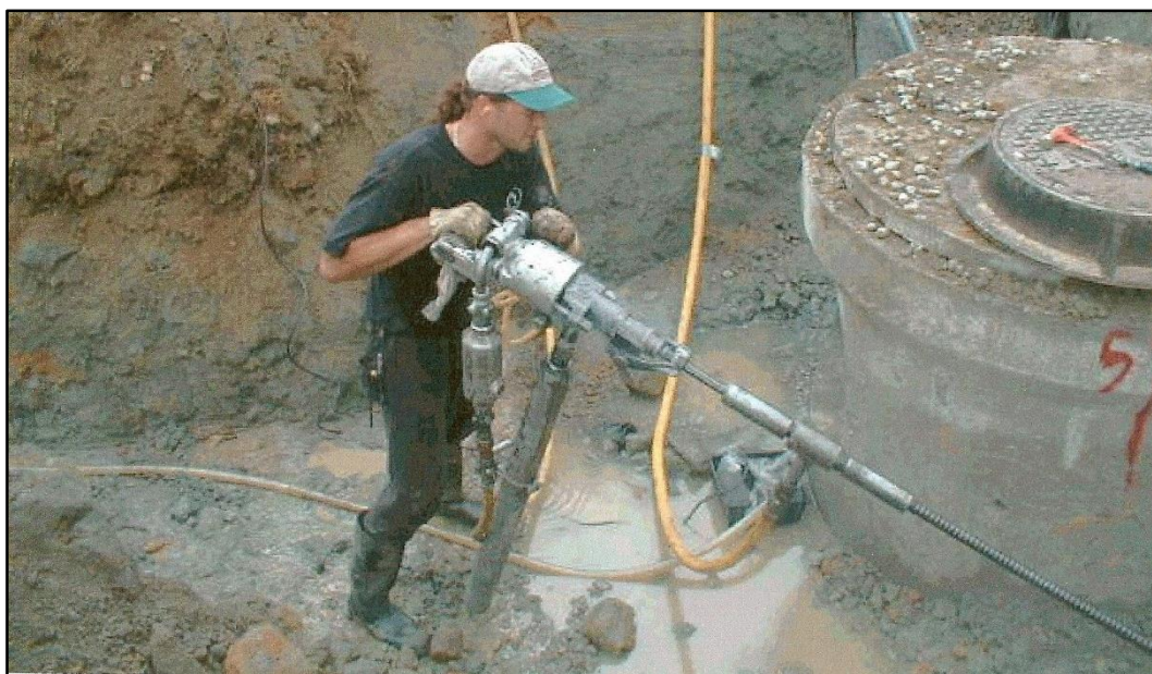
شکل ۶: جایگزاری المان میله‌ای در حفره
