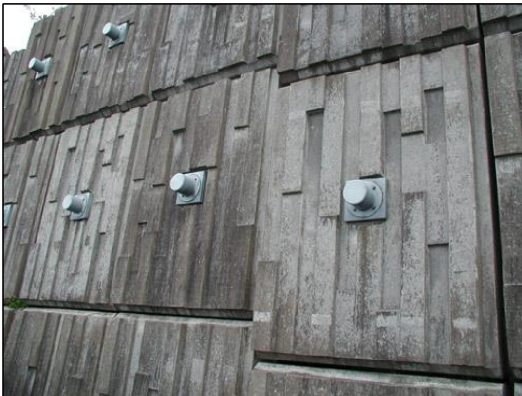
شکل ۲۰: استفاده از انکراژ و بلوک
