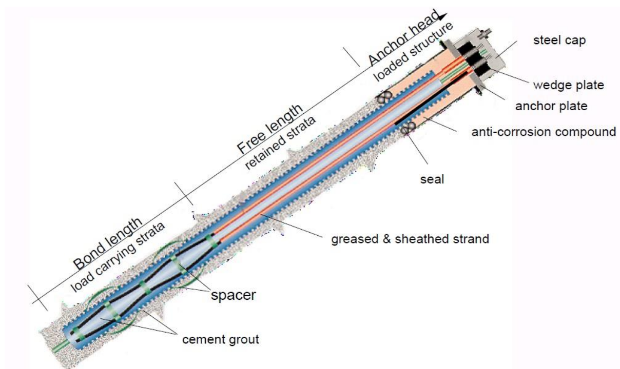
شکل ۲: اجزای سیستم انکراژ
